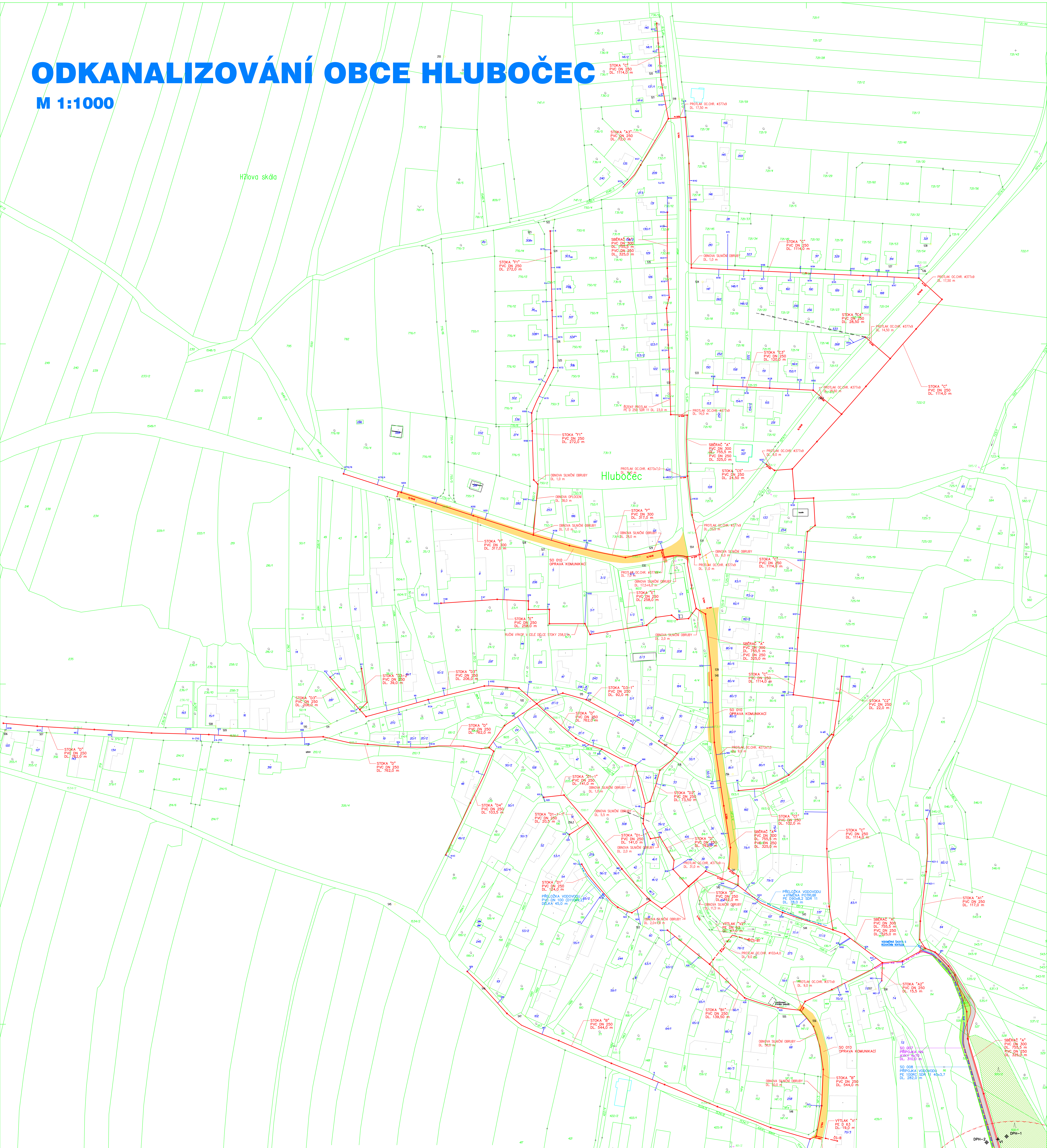
Obec Hlubočec - stoková síť splaškové kanalizace
